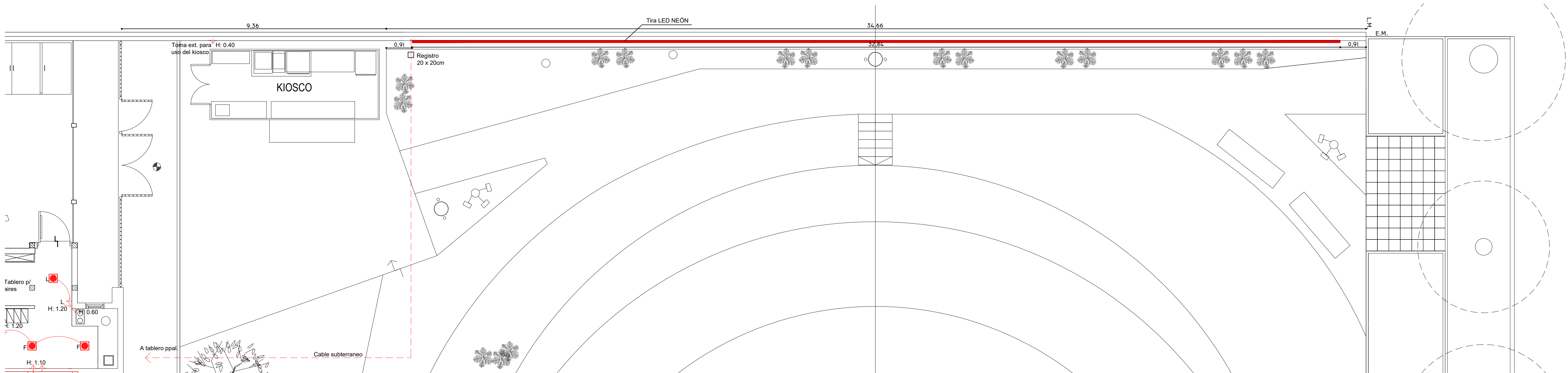
PLANTA ELECTRICIDAD MEDIANERA
