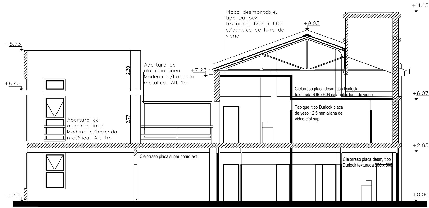
Corte A-A
