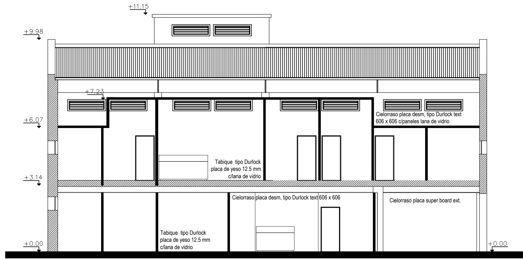
Corte D-D
