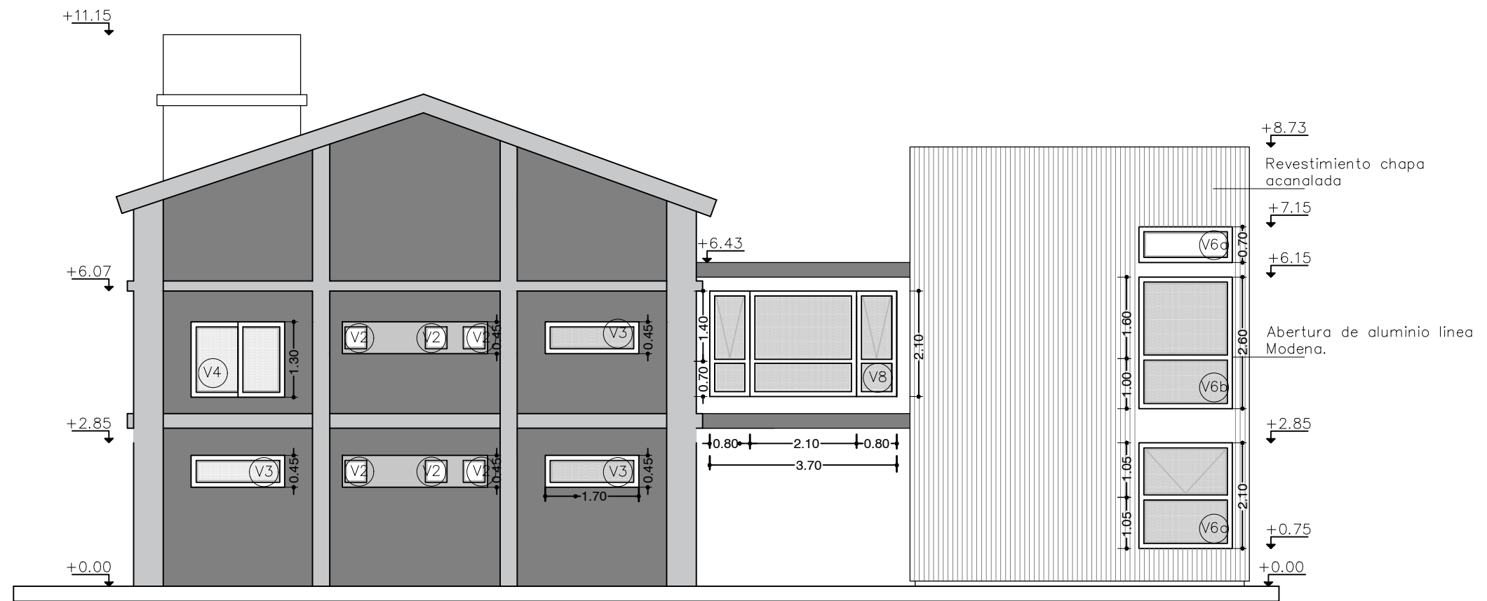
Vista Lateral
